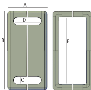
Front/Rückplatte / geteilt
